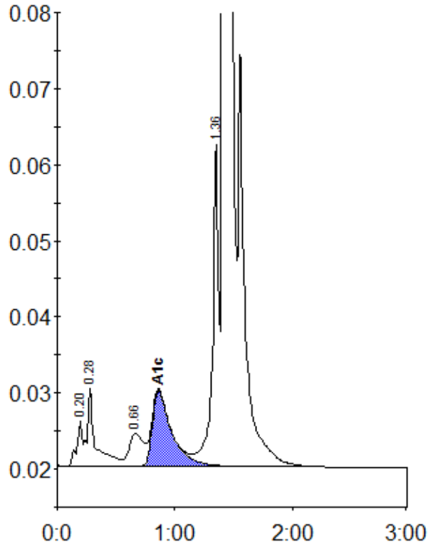
Peak table - ID: 10550276
